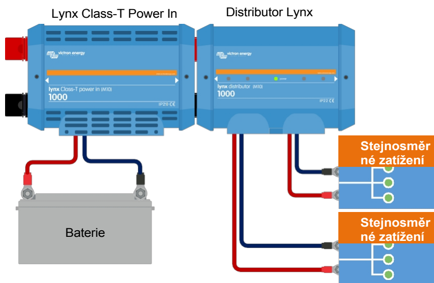
Systém s napájecím vstupem Lynx třídy T a rozdělovačem Lynx
