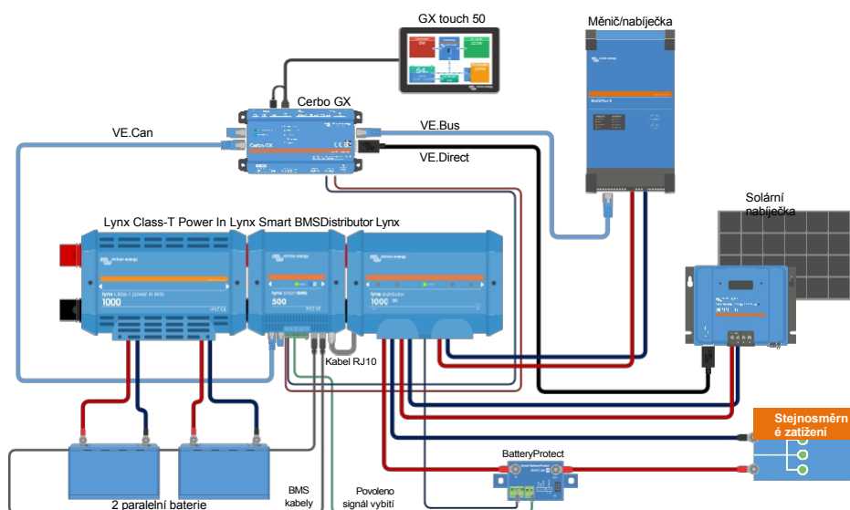
Systém s napájecím zdrojem Lynx Class-T, dvěma lithiovými inteligentními bateriemi, inteligentní řídicí jednotkou Lynx Smart BMS a rozdělovačem Lynx.
