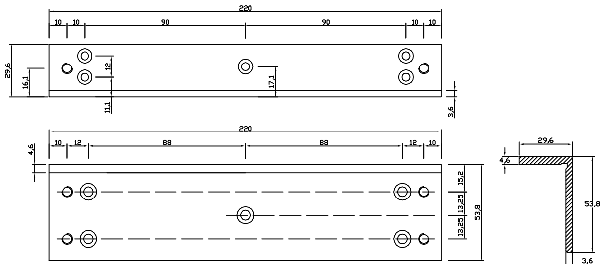
„L“ konzole MAG-280 outdoor
