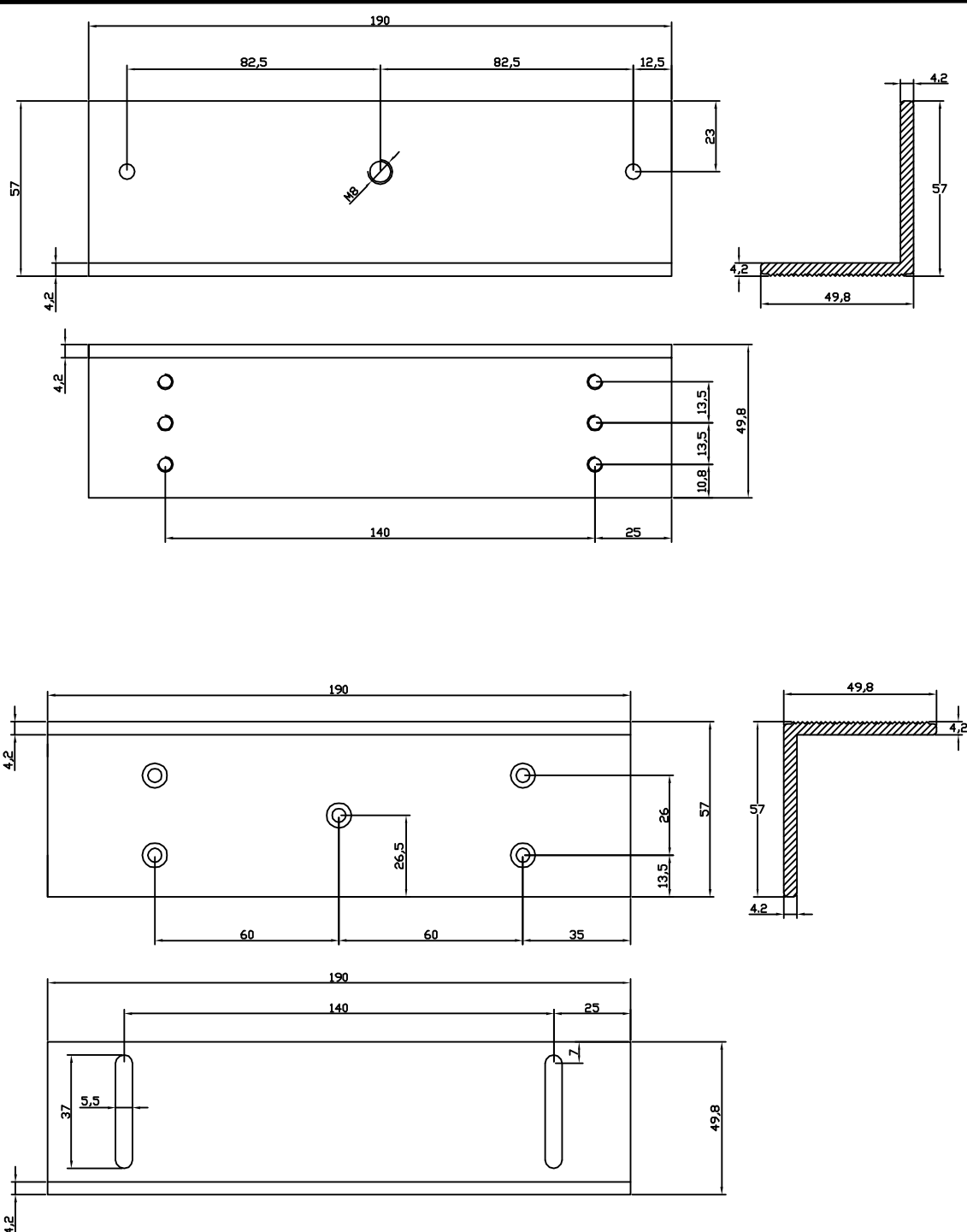
„Z“ konzole MAG-280 outdoor
