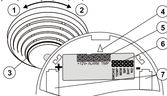
Obrázek 1: 1 – otevření detektoru; 2 – zavření detektoru; 3 – optická signalizace stavu; 4 – orientační šipka pro nasazení; 5 – svorkovnice; 6 – konfigurační propojky; 7 – prostor pro vložení baterií
