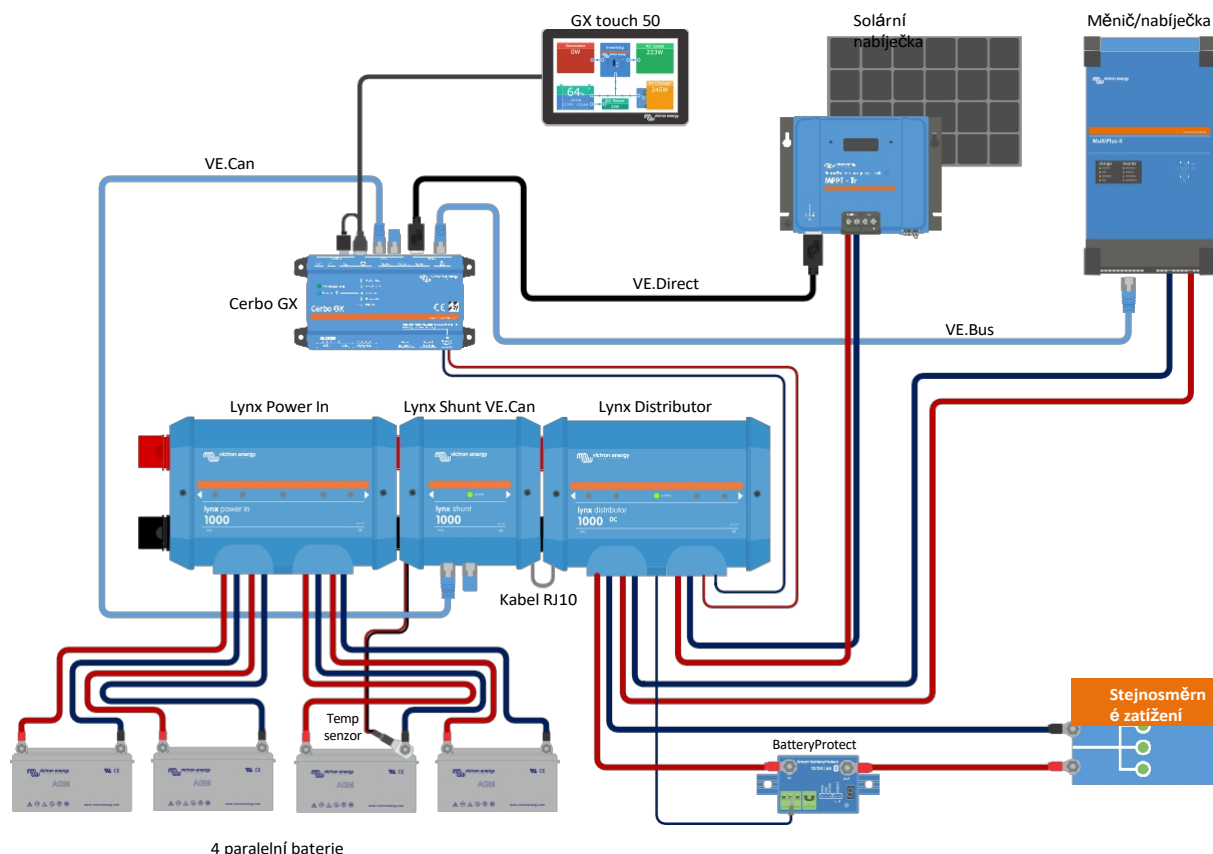
Systém s bočником Lynx VE.Can, olověnými akumulátory, bočником Lynx VE.Can a rozdělovačem Lynx.
