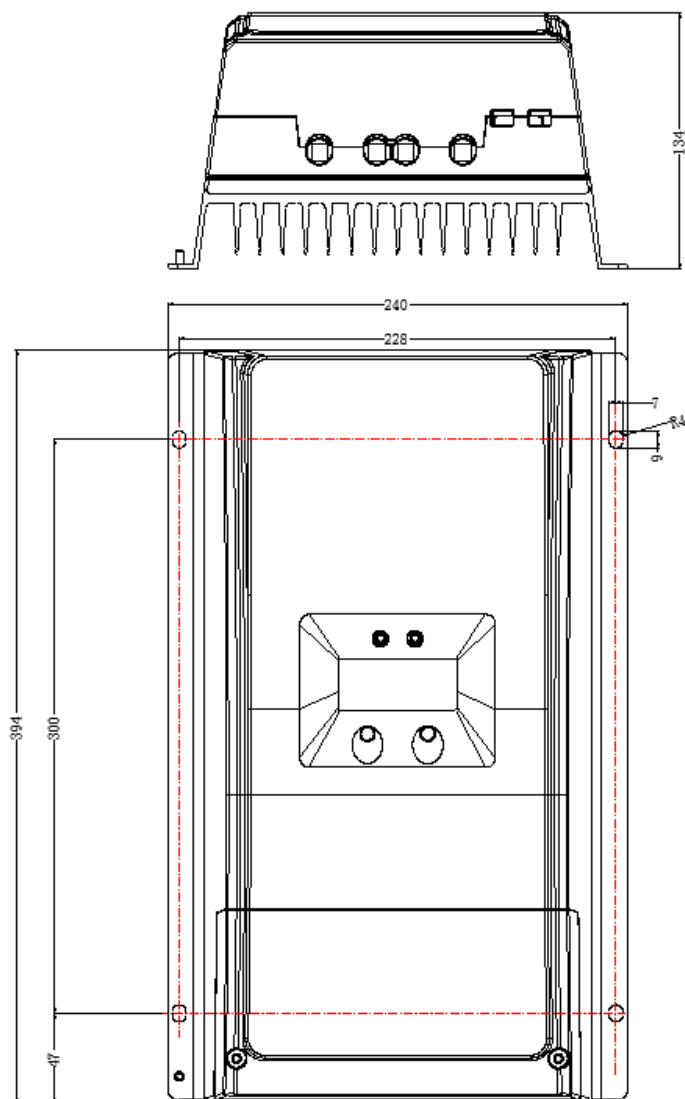
Tracer8415/8420AN Rozměry (Jednotka: mm)
