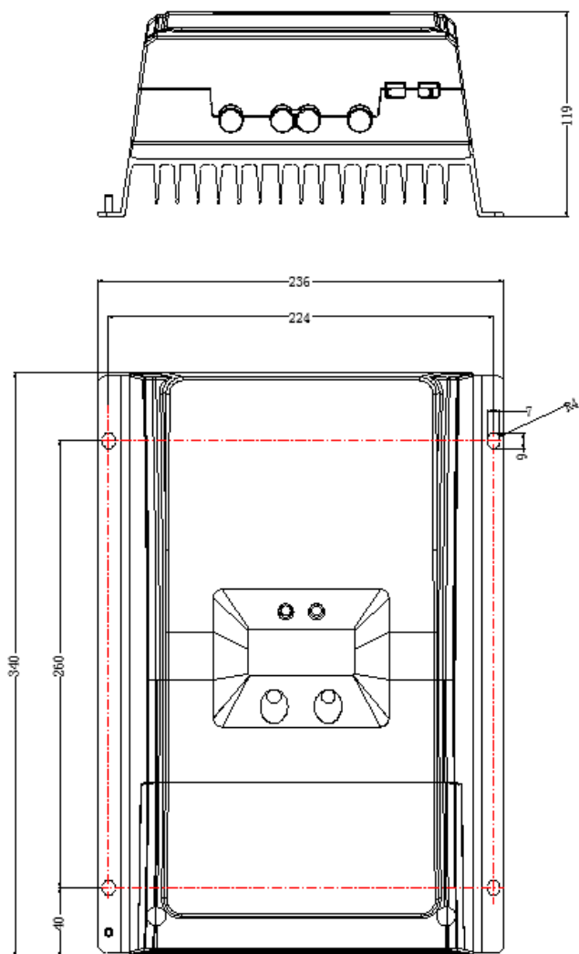
Tracer6210/6415/6420AN Rozměry (jednotka: mm)
