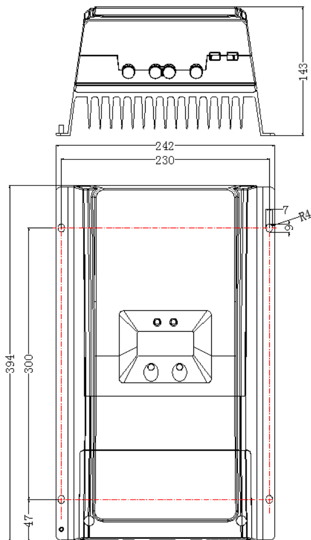
Tracer10415/10420AN Rozměry (Jednotka: mm)
