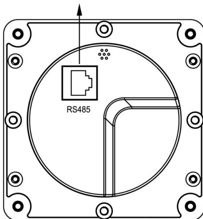
Zadní pohled
